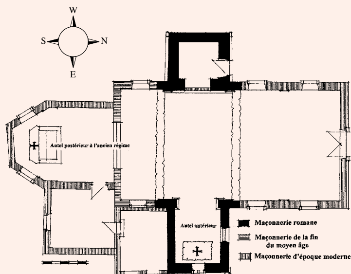
Plans superposés des différentes constructions de l'église
